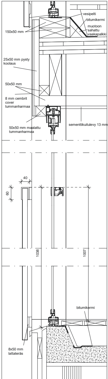
DET5 PARVEEKEN ETUOSA
