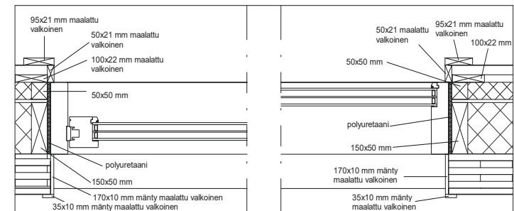
LIUKUOVEN VAAKALEIKKAUS
