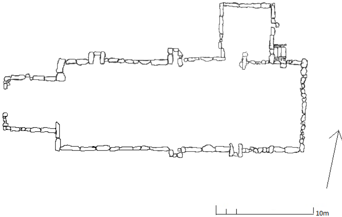
Kuva 2. Hailuodon kirkon pohjapiirros. Muokattu J. Okkosen kenttäpiirroksesta. 30
